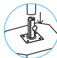
Schraubbare Rohrhülse mit Spreizfunktion
