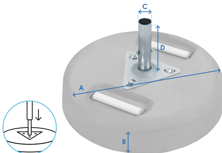
Aufsatzrohr Standard
