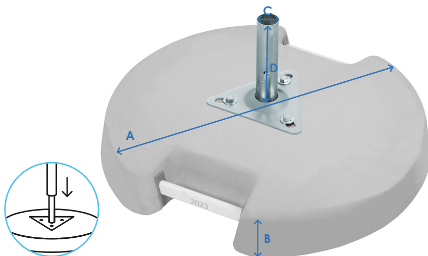
Aufsatzrohr Standard
