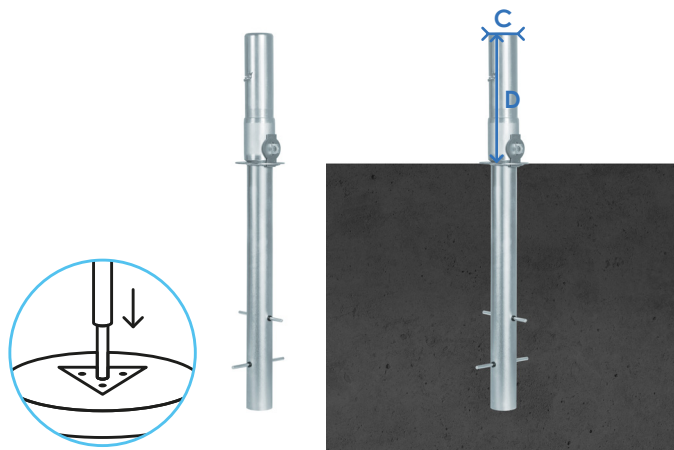
Aufsatzrohr Standard
