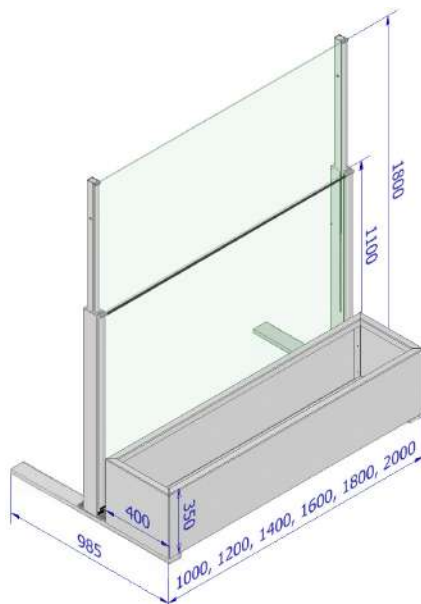
Wind Barrier mit Aluminiumtopf
