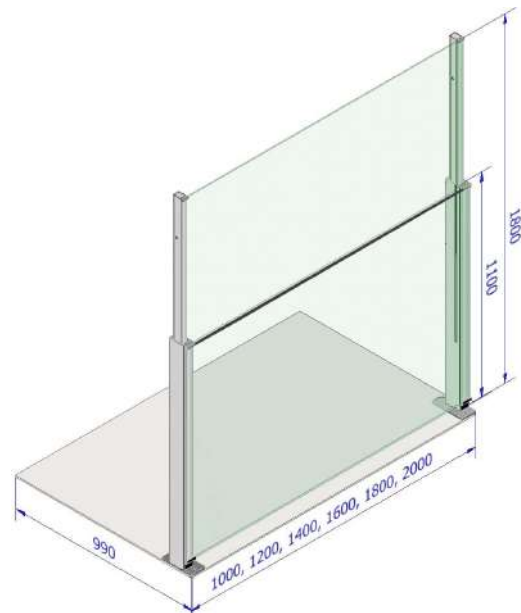
Wind Barrier mit Stahlstnde
