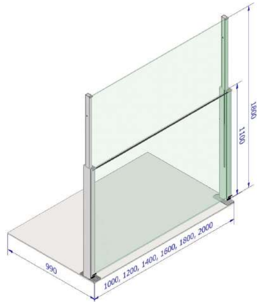
Wind Barrier mit Stahlstände
