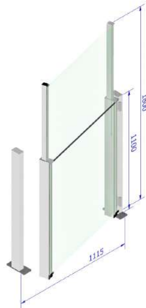
Wind Barrier mit Stahlstände
